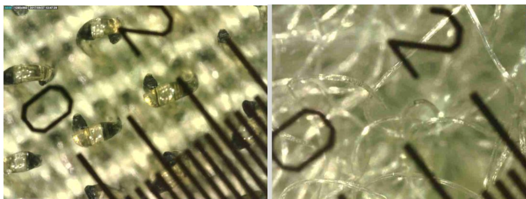
Suchý zip pod mikroskopem – vzdálenost na pravítku jsou milimetry
